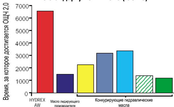
Сравнительное испытание на окисление по стандарту ASTM D943 (ISO 46)
